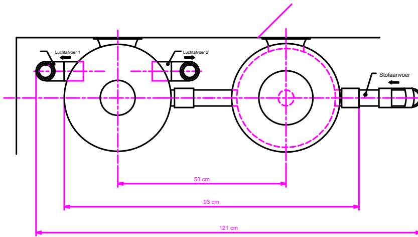
Bovenaanzicht
