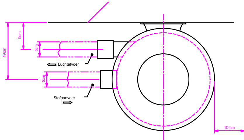
Bovenaanzicht MK 23 stofzuigunit
